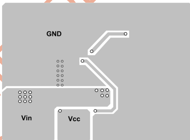
Bottom Layer
