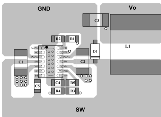
Top Layer
