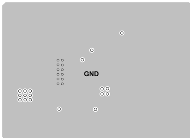
Inner Layer1
