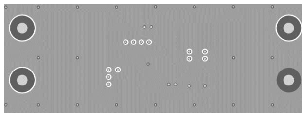
Inner 1 Layer
