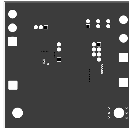
Mid Layer 1
