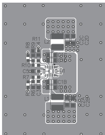
Top Layer
