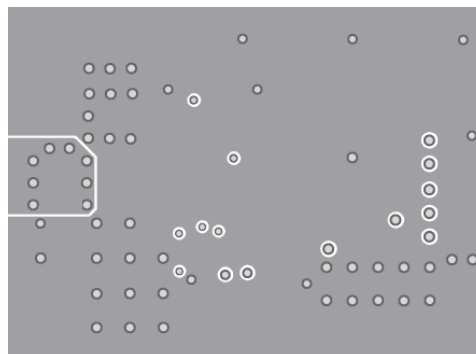
Bottom Layer
