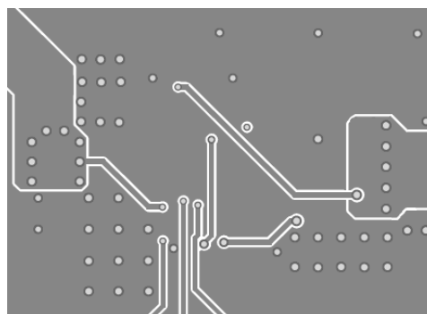
Inner Layer 2
