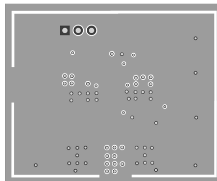
Inner Layer 1
