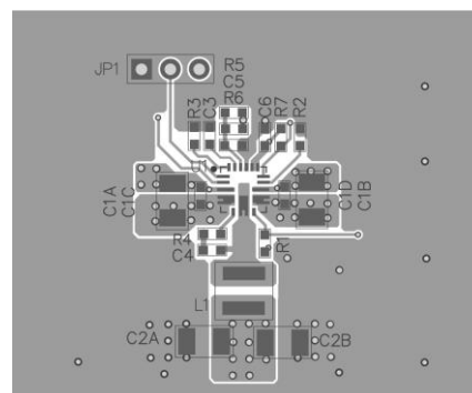
Top Layer
