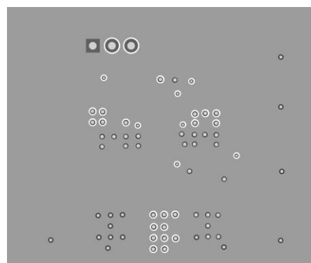
Bottom Layer
