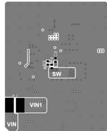
Bottom Layer
