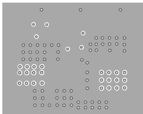
Bottom Layer
