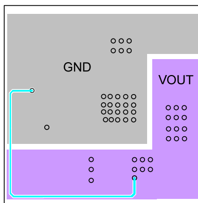
Bottom Layer
