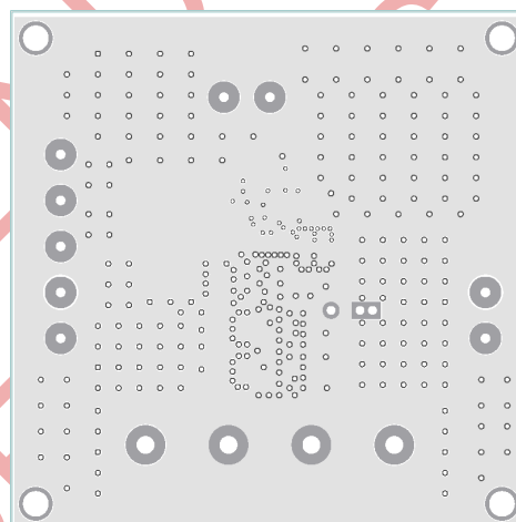
Inner2 Layer
