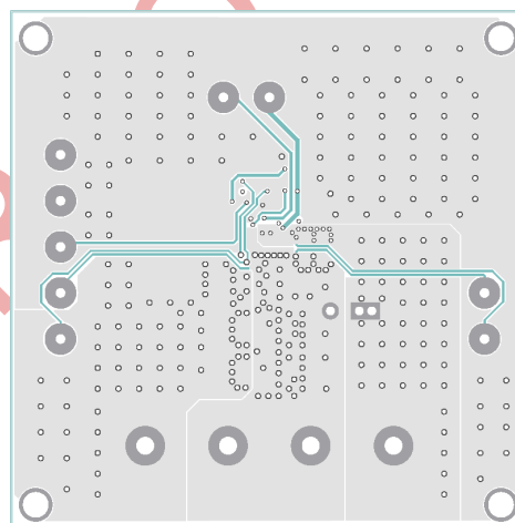
Bottom Layer
