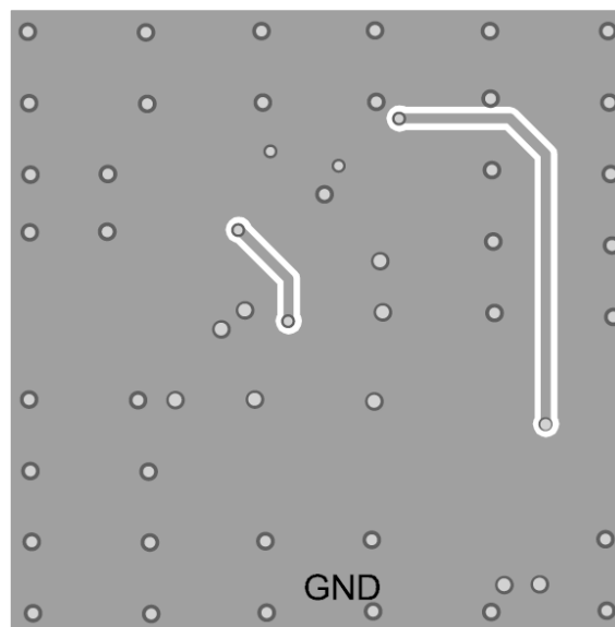
Bottom Layer
