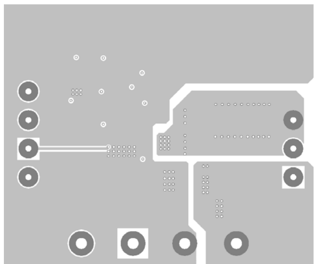
Bottom Layer
