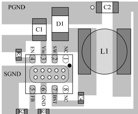
Top Layer
