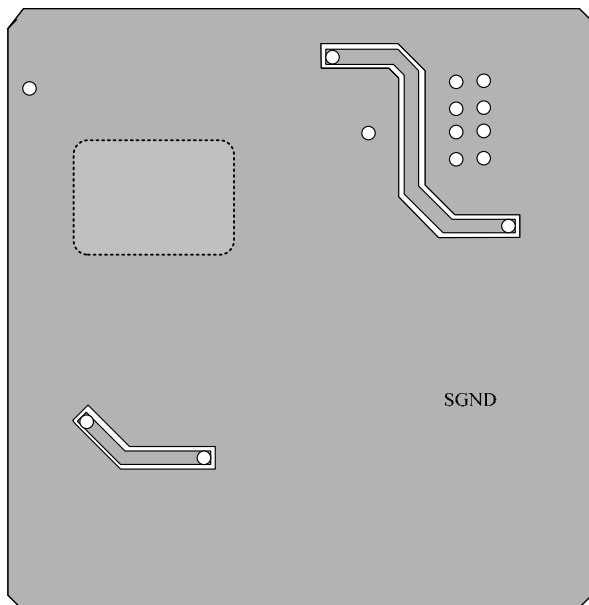
Bottom Layer
