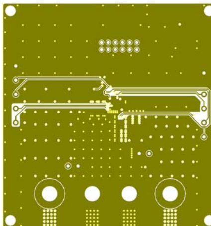
Figure 4— Inner Layer 2
