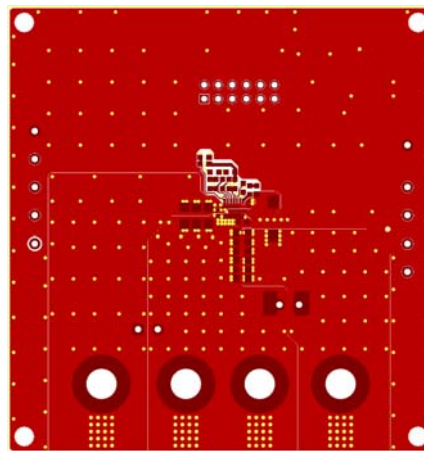
Figure 2—Top Layer
