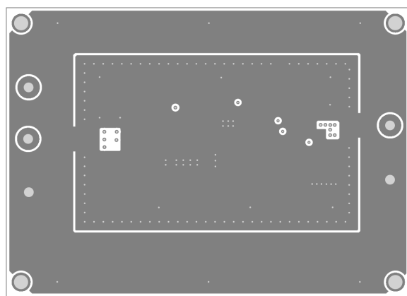
Figure 1—Inner1 Layer
