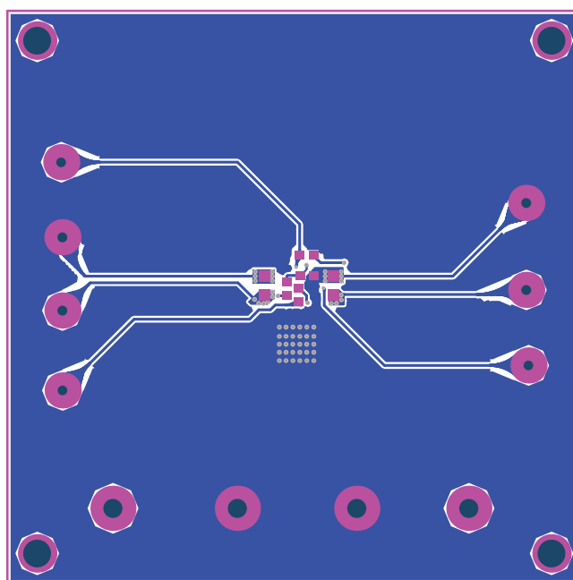
Figure 5—Bottom Layer
