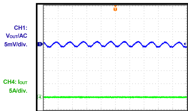
Vo Ripple
