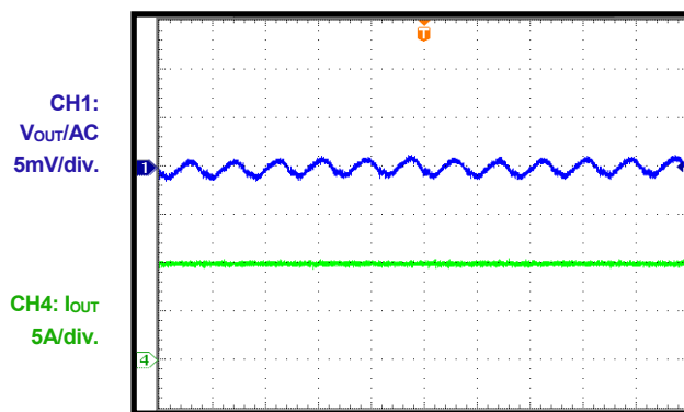
Vo Ripple
