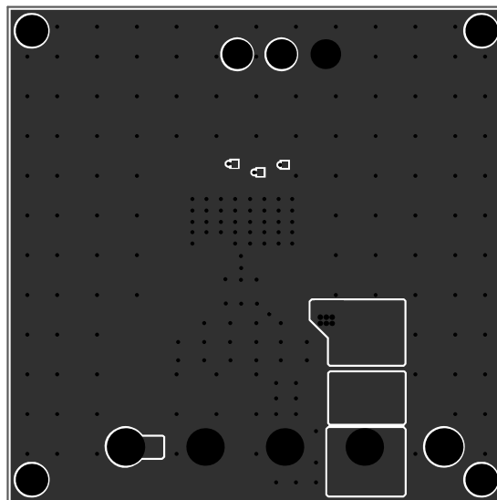
Figure 2—Bottom Layer
