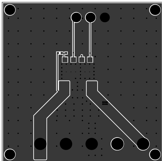
Figure 1—Top Layer
