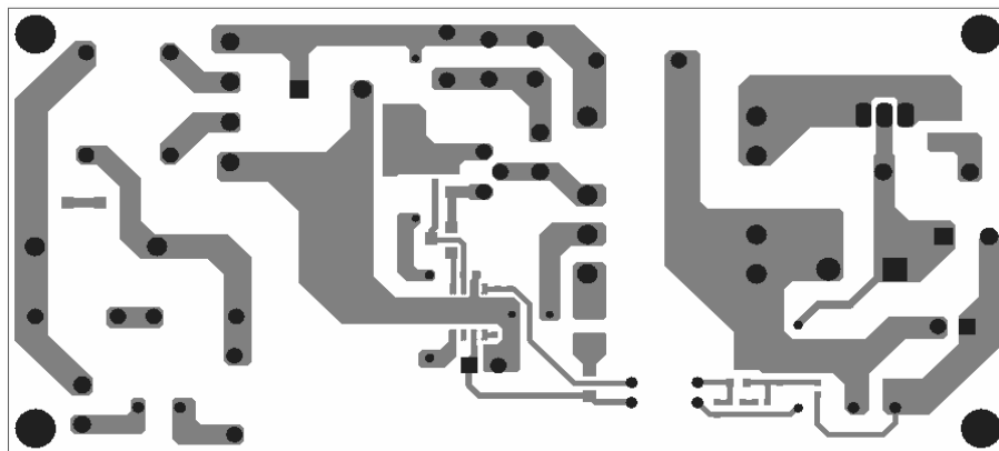
Figure 3 — Bottom Layer
