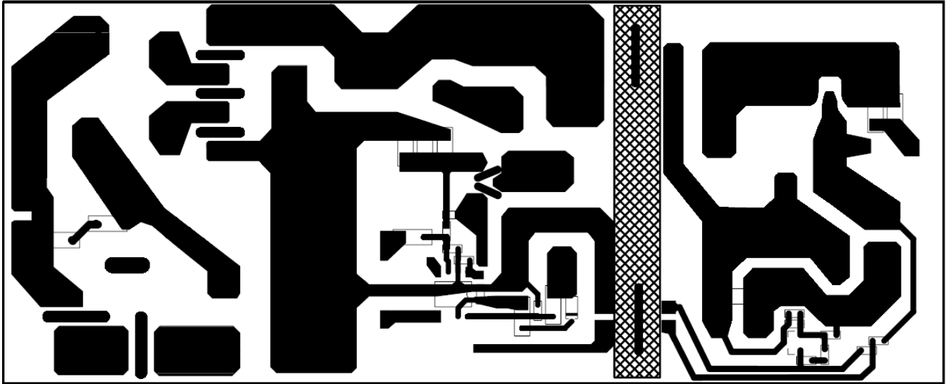
Figure 3 — Bottom Layer
