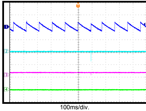
Input/Output Ripple
