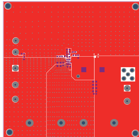
Figure 2—Top Layer
