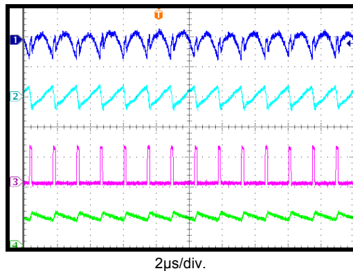
Input/Output Ripple
