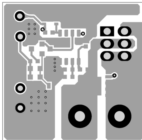
Figure 2—Top Layer
