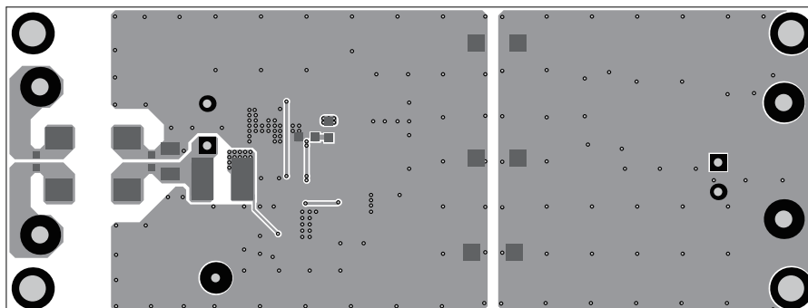
Figure 4—Bottom Layer
