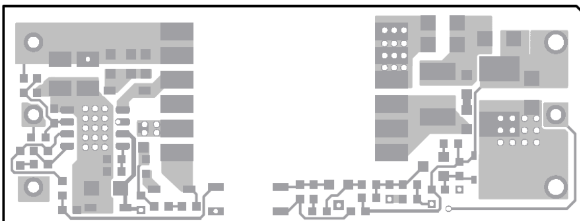
Figure 1—Top Layer
