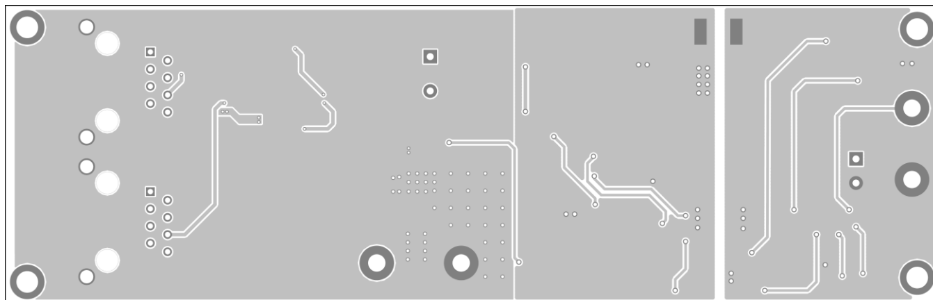
Figure 3—Bottom Layer
