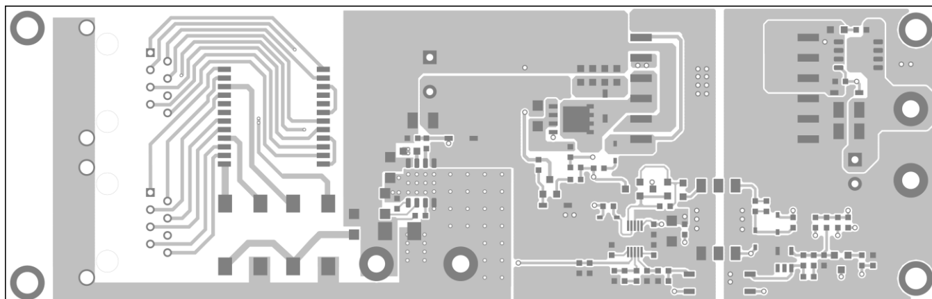
Figure 2—Top Layer
