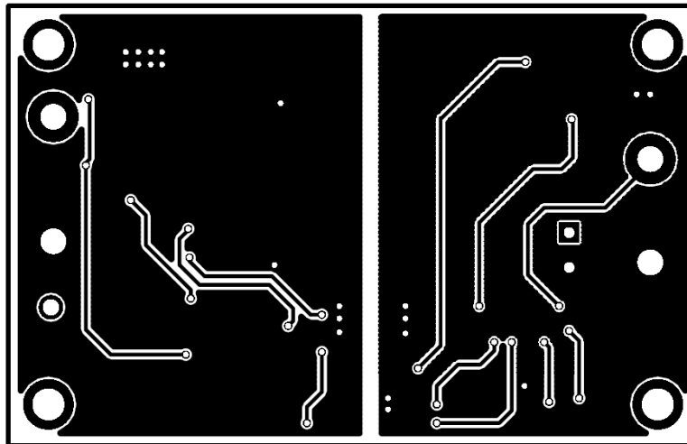
Figure 3—Bottom Layer
