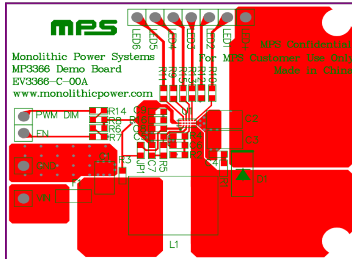
Figure 1—Top Layer
