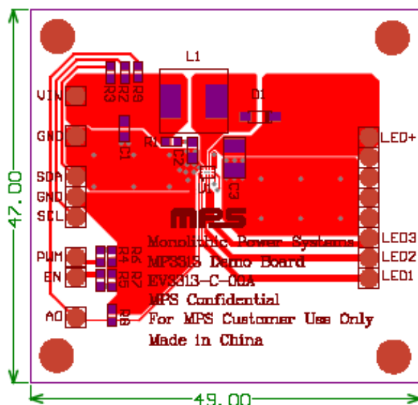
Figure 1—Top Layer
