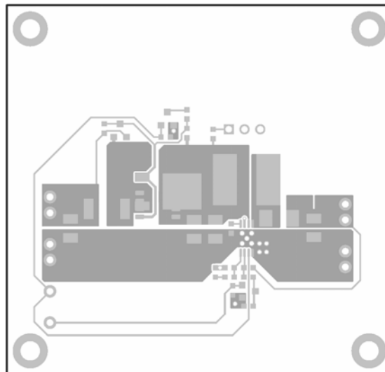
Figure 2—Top Layer
