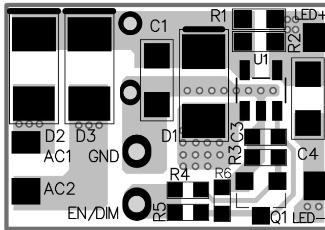
Figure 1—Top Layer
