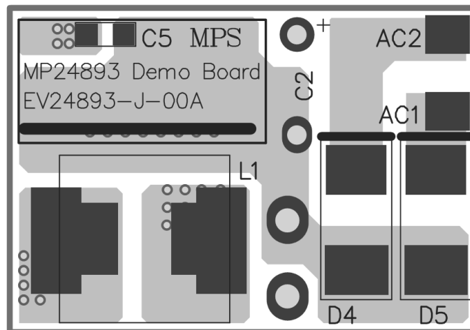
Figure 2—Bottom Layer
