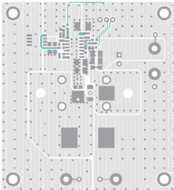
Figure 3—Top Layer
