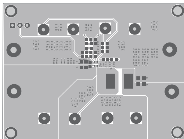
Figure2: Top Layer
