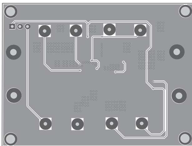
Figure3: Bottom Layer
