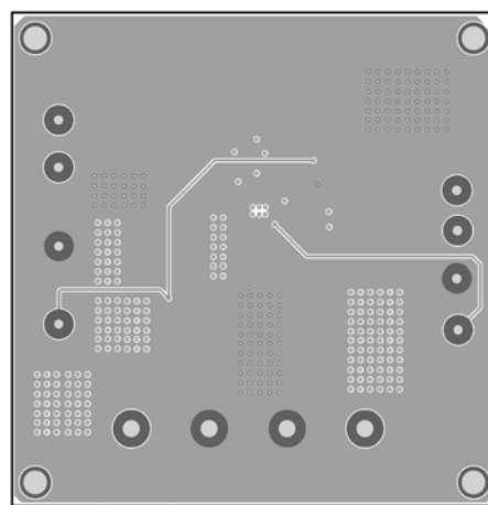
Figure 4— Inner 2 Layer
