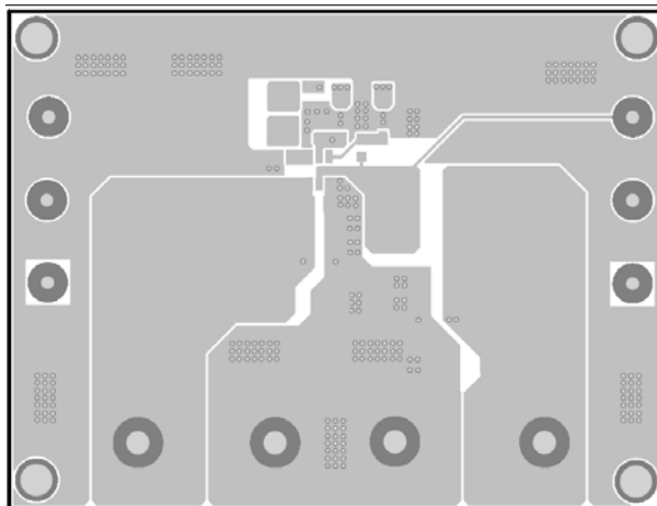
Figure 2—Top Layer
