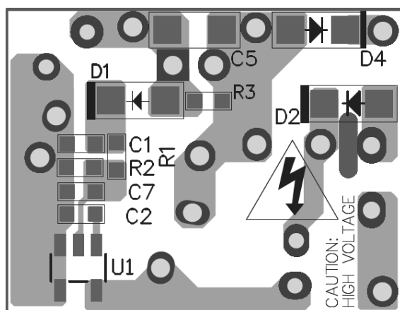
Figure 3—Bottom Layer
