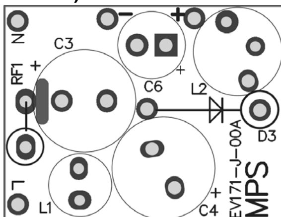
Figure 2—Top Layer
