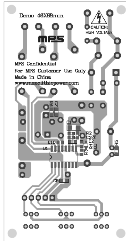
Figure 3—Bottom Layer
