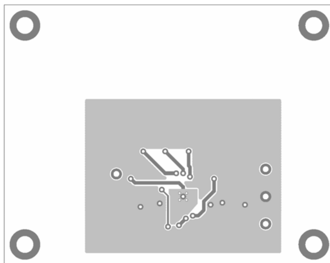
Figure 3—Bottom Layer
