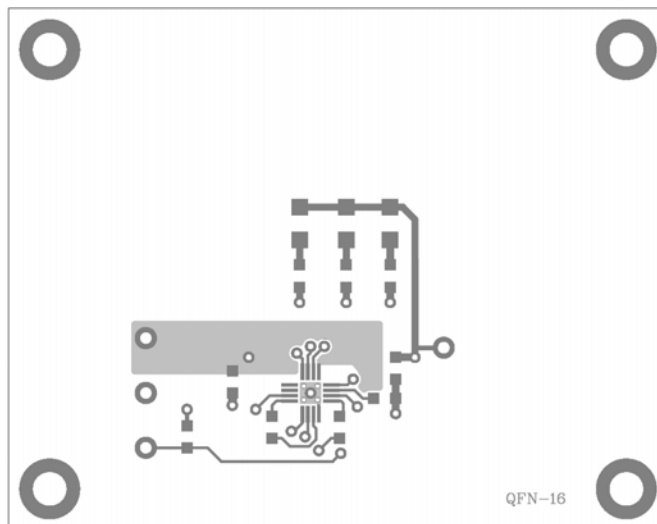
Figure 2—Top Layer
