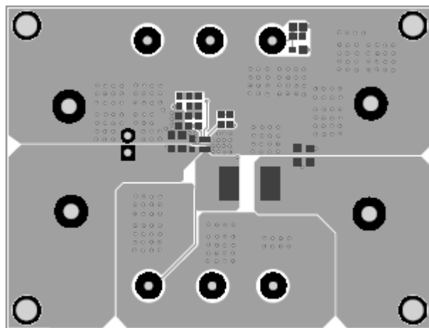
Figure2: Top Layer
