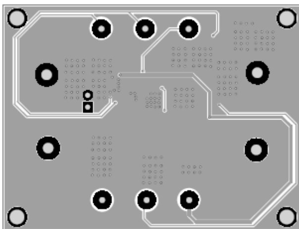
Figure3: Bottom Layer
