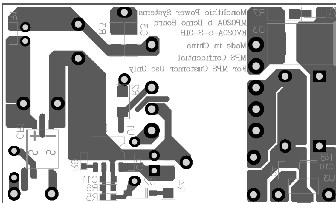
Figure 3—Bottom Layer
