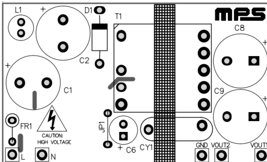
Figure 2—Top Layer
