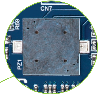
Figure 15-1: Buzzer module
