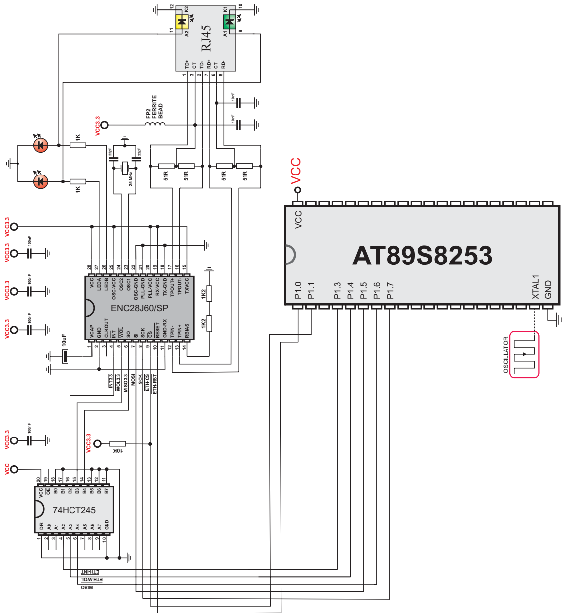
6.12. SPI Ethernet
