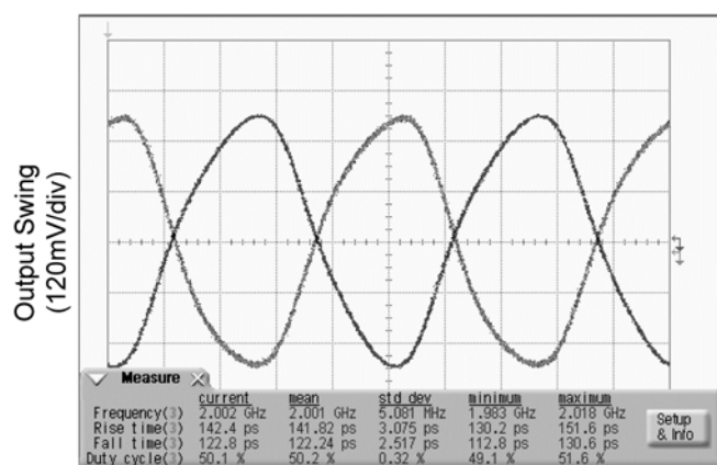
2GHz Output
