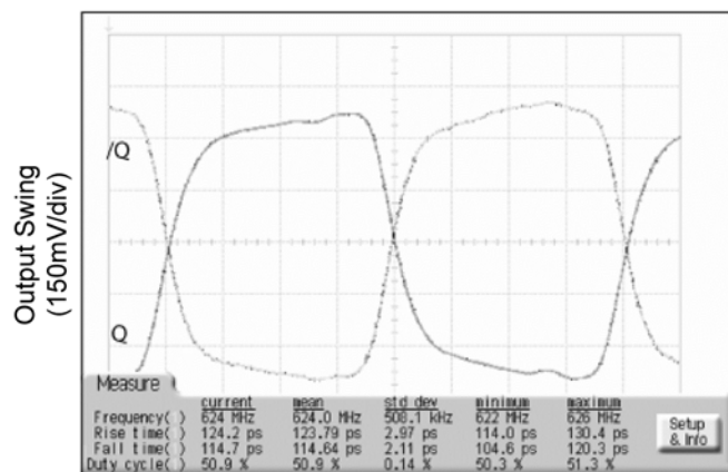
155MHz Output
