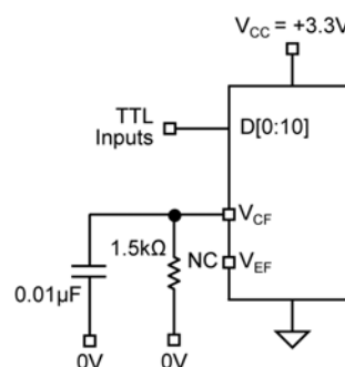
Figure 14. V_{CF}/V_{EF} Biasing for LVTTTL Control (D) Input
