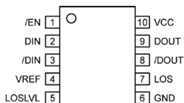
10-Pin EPAD-MSOP (K10-2)
