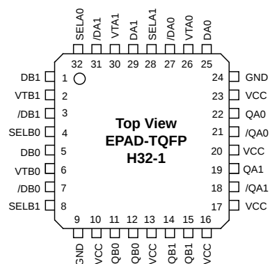
32-Pin EPAD-TQFP (H321)
