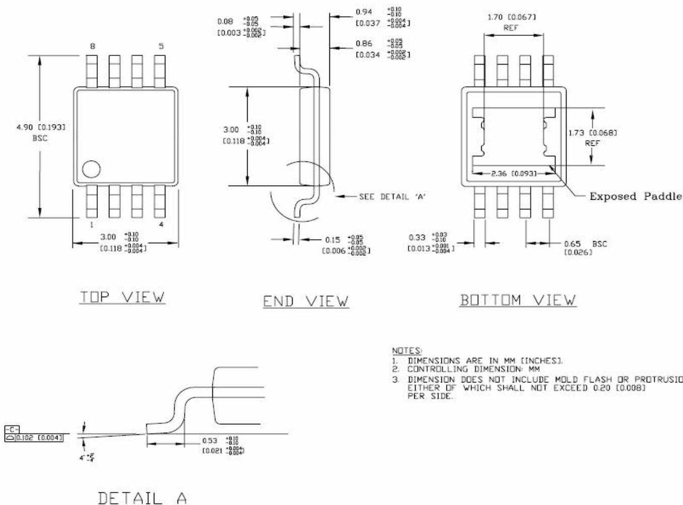
8-Pin ePAD MSOP (MME)
