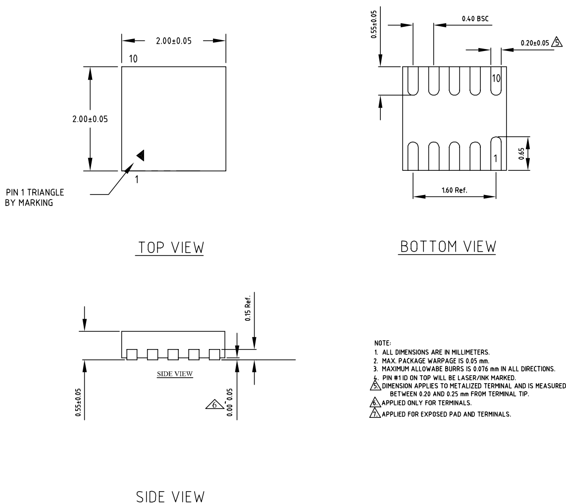
10-Pin 2mm x 2mm Thin MLF ® (MT)
