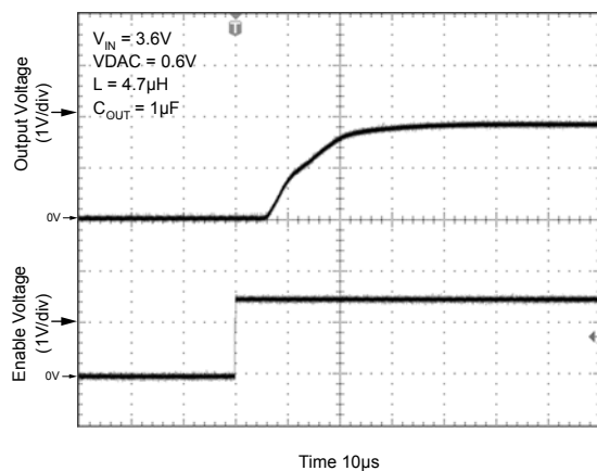
Enable Transient
