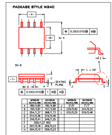
SO-8
